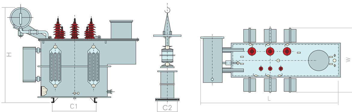
SZ9-800~31500/35变压器
